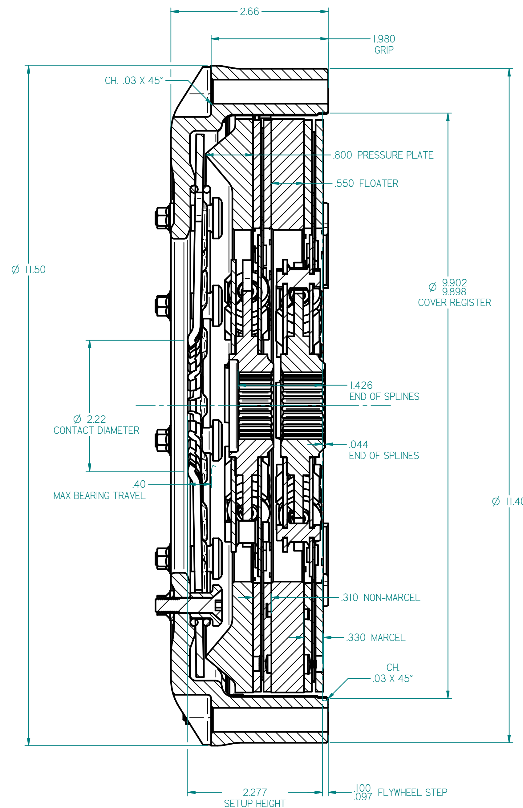
SECTION A-A
