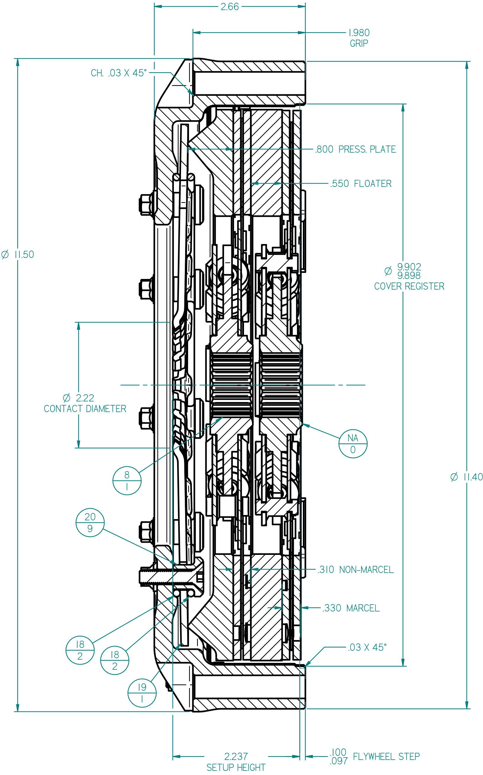
SECTION A-A
